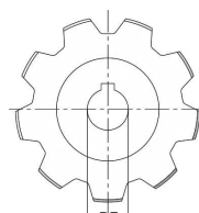
Solid Sprocket
