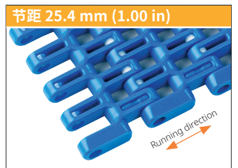
uni SNB M2 强度指数 (聚甲醛)
