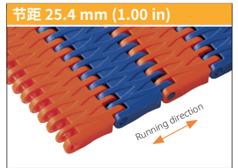
uni JCB Y 强度指数 (聚甲醛)
